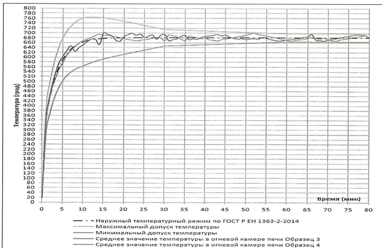
Рисунок 9. График температурного режима в огневой камере печи при испытании образцов №№ 3, 4 по ГОСТ Р ЕН 1363-2-2014 (Наружный температурный режим)
