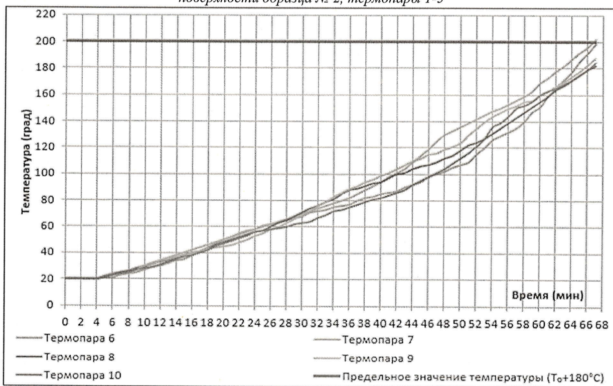
Рисунок 7. График локальных значений и среднего значения температуры на необогреваемой поверхности образца № 2, термопары 6-10
