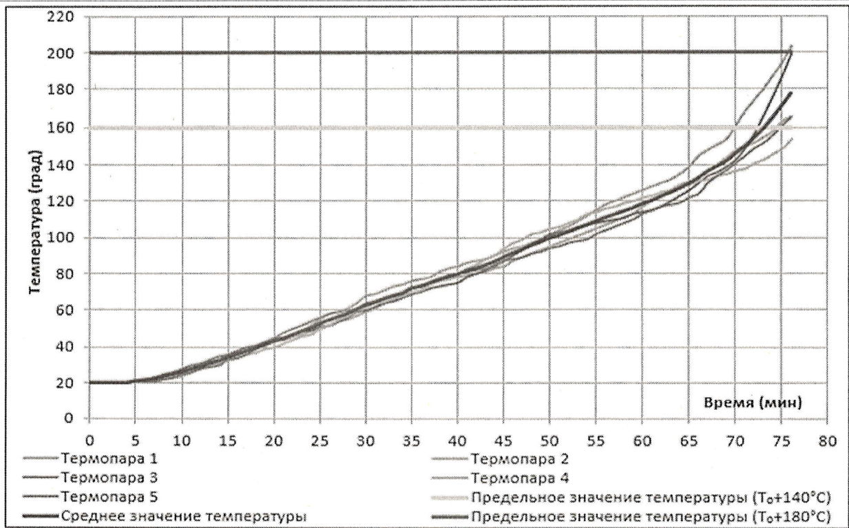
Рисунок 6. График локальных значений и среднего значения температуры на необогреваемой поверхности образца № 2, термопары 1-5
