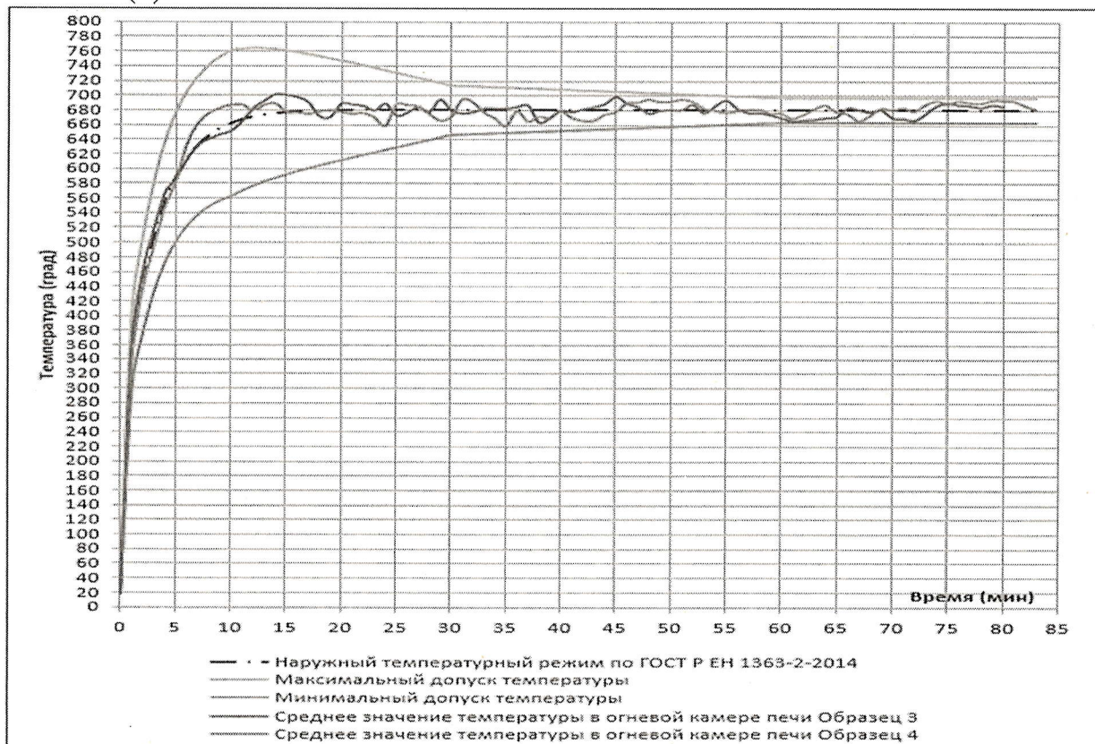
Рисунок 9. График температурного режима в огневой камере печи при испытании образцов №№ 3, 4 по ГОСТ Р ЕН 1363-2-2014 (Наружный температурный режим)
