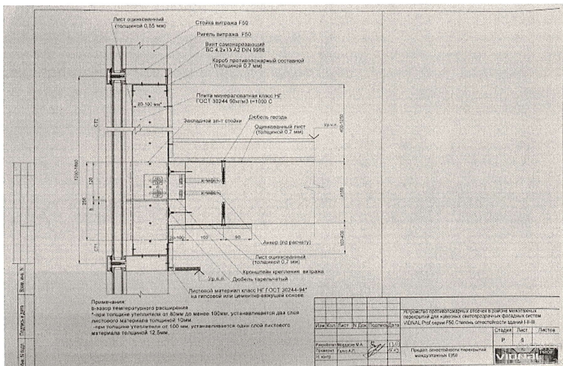
Рисунок 1 – сечение междуэтажного пояса
