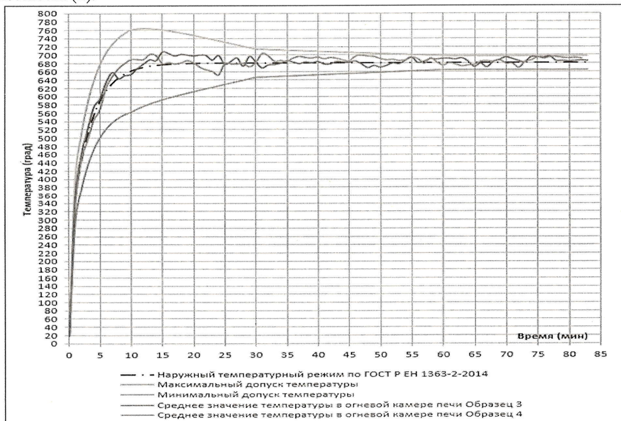
Рисунок 9. График температурного режима в огневой камере печи при испытаниях образцов №№ 3, 4 по ГОСТ Р ЕН 1363-2-2014 (Наружный температурный режим)
