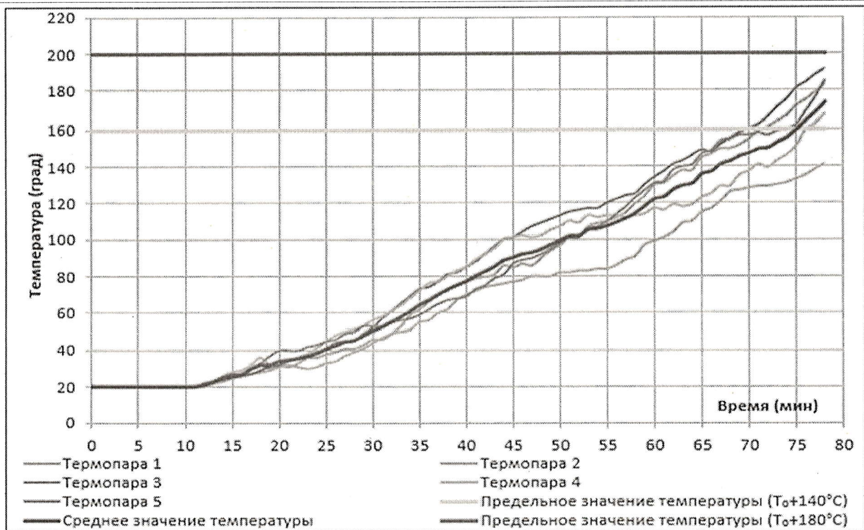
Рисунок 6. График локальных значений и среднего значения температуры на необогреваемой поверхности образца № 2, термопары 1-5
