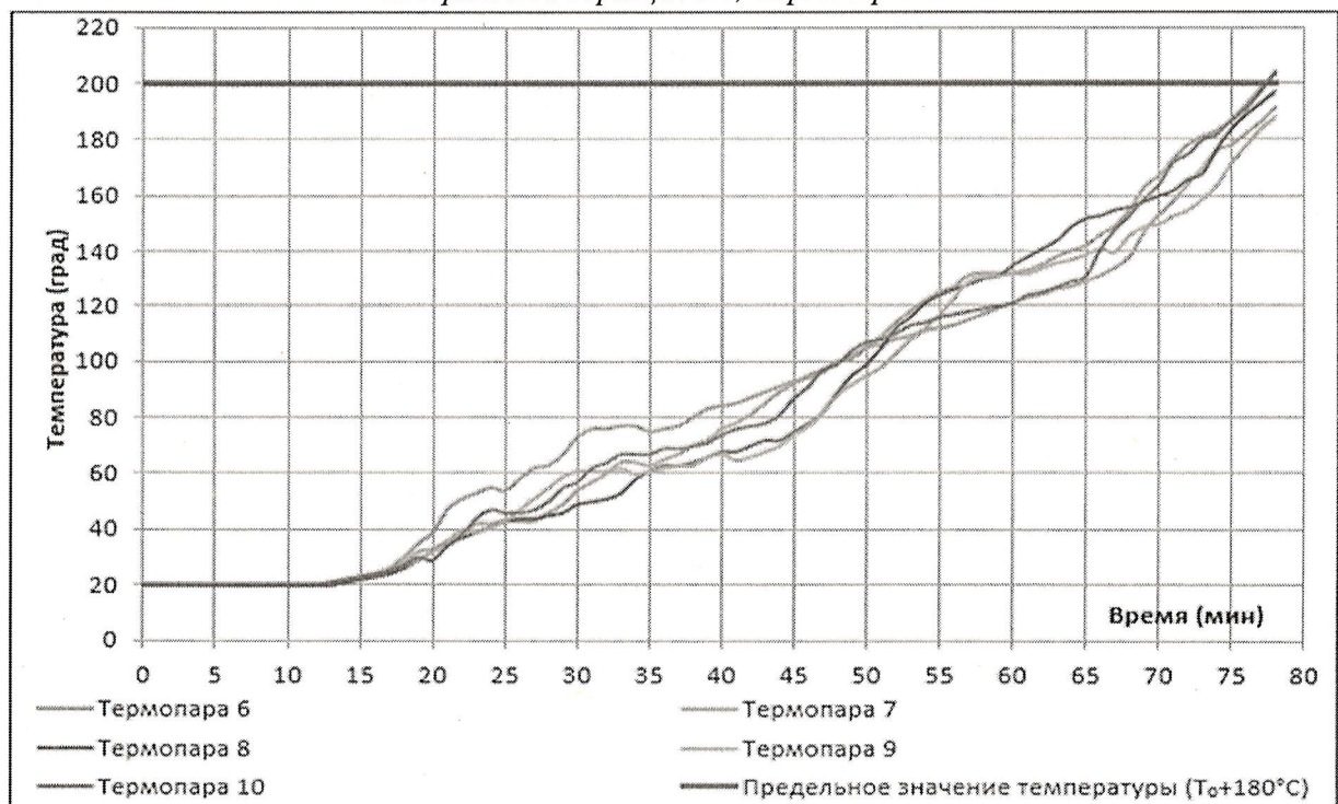
Рисунок 7. График локальных значений и среднего значения температуры на необогреваемой поверхности образца № 2, термопары 6-10
