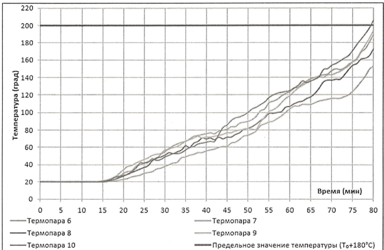
Рисунок 5. График локальных значений и среднего значения температуры на необогреваемой поверхности образца № 1, термопары 6-10
