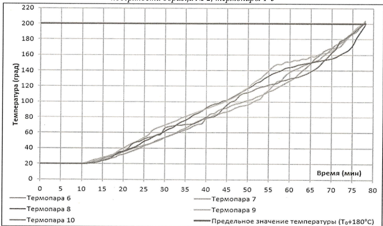
Рисунок 7. График локальных значений и среднего значения температуры на необогреваемой поверхности образца № 2, термопары 6-10
