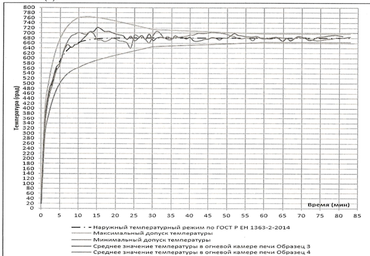
Рисунок 9. График температурного режима в огневой камере печи при испытании образцов №№ 3, 4 по ГОСТ Р ЕН 1363-2-2014 (Наружный температурный режим)
